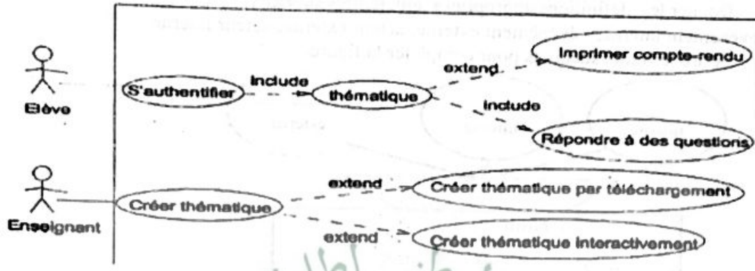
FIGURE 1 – Diagramme de cas d'utilisation
